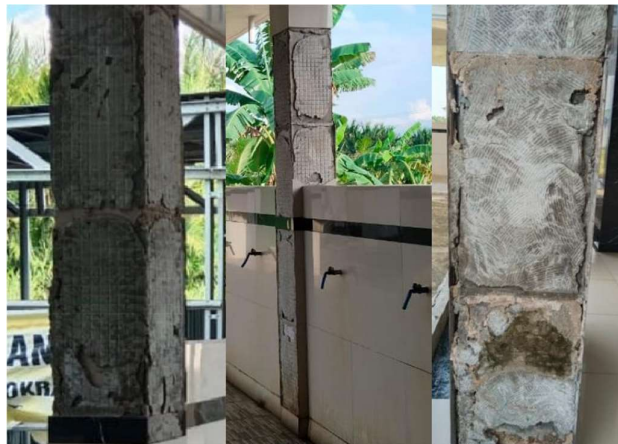
Gambar 20. Bidang rekatan yang tidak penuh dengan pasta perekat
