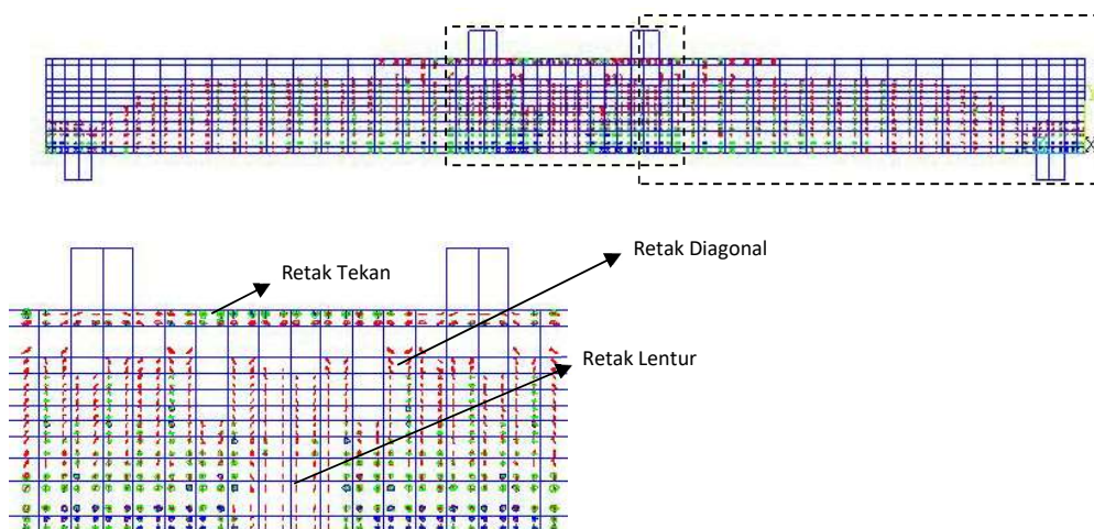
Gambar 1. Pola Retak Ultimit Balok BEV
