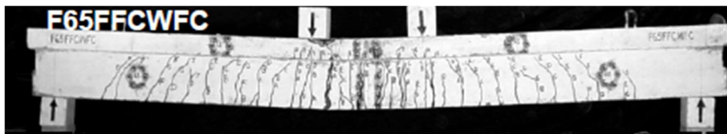
Gambar 1. Pola Retak Balok Eksperimen
